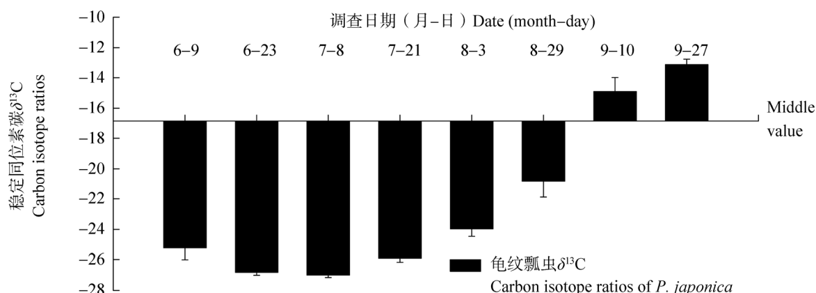
图 3 2010 年不同时期棉花和玉米农田景观系统中龟纹瓢虫 \delta^{13}\text{C} 值变化 Fig. 3 Carbon isotope ratios of Propylea japonica adults collected from maize patches in 2010
